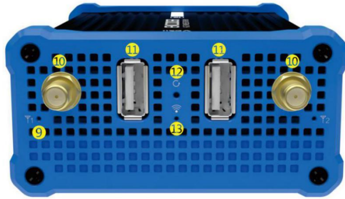
9、WiFi 天线增益灯 10、WiFi 天线接口 11、USB 扩展接口 12、reset 按钮 13、WiFi 状态灯
